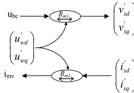
Fig. 5.11. GIC du convertisseur moyen.
