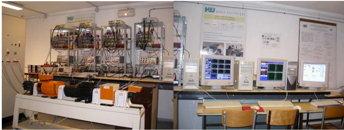
Fig. 8.3. Plate-forme expérimentale.
