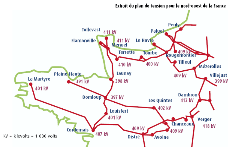
Fig. 2.21. Exemple de plan de tension et de points pilotes [RTE02].
