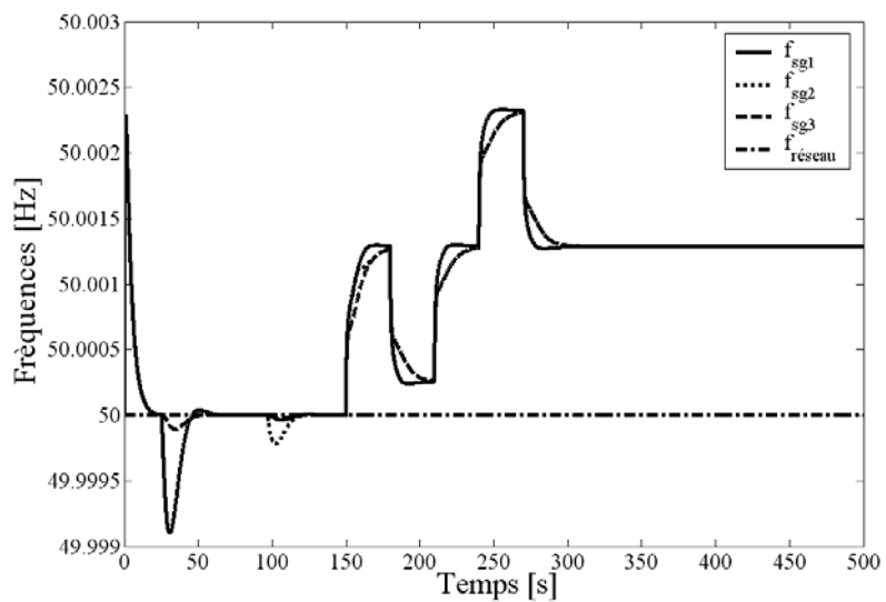
Fig. 7.12. Fréquences des sources.
