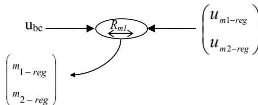
Fig. 6.28. GIC de la commande du convertisseur.
