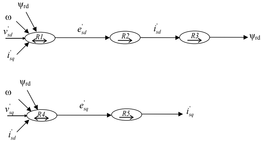
Fig. 5.4. GIC de la machine asynchrone.
