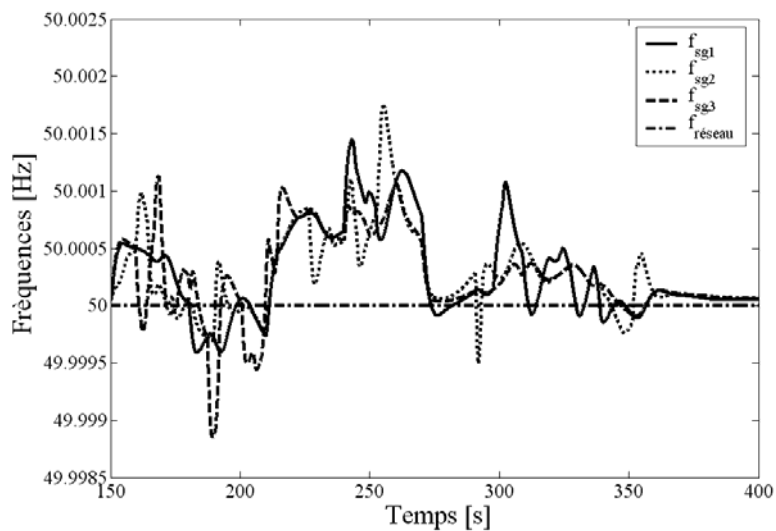
Fig. 7.47. Fréquences des systèmes de génération pendant l'îlotage.
