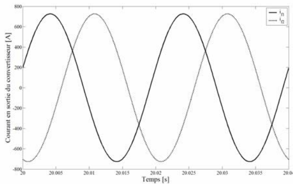
Fig. 6.43. Courants i_{f1} , i_{f2} .
