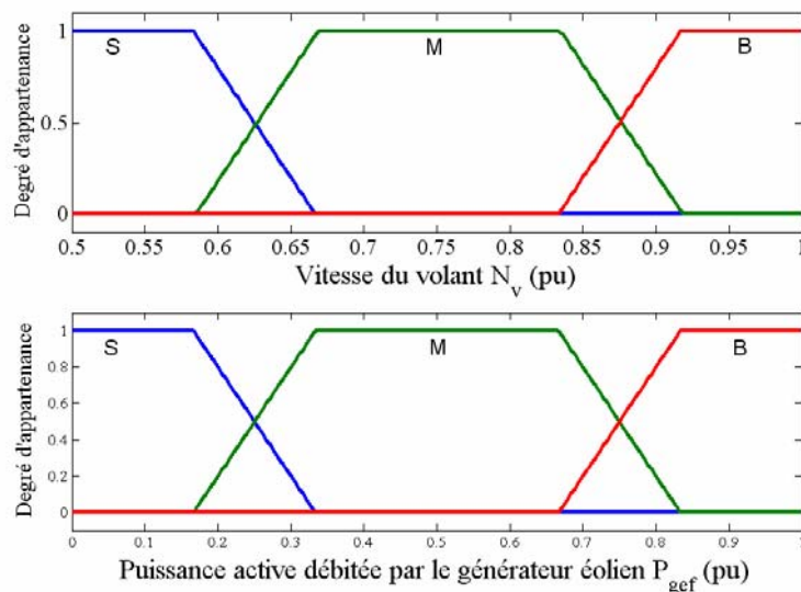
Fig. 7.30. Fonctions d'appartenance des variables d'entrées.
