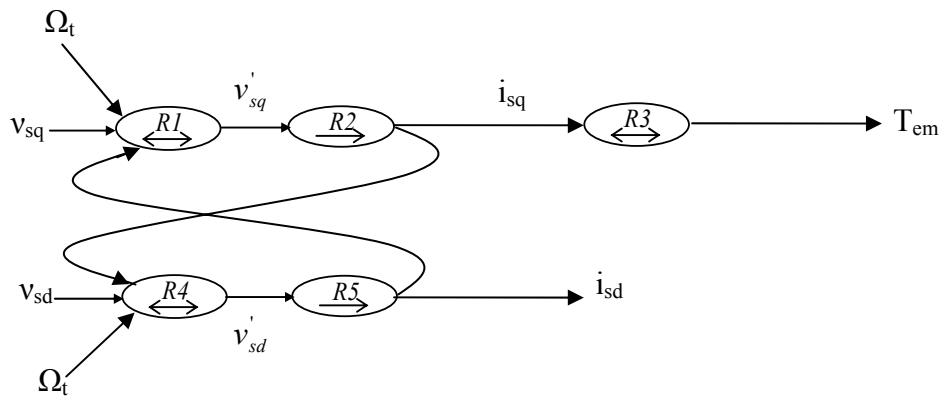
Fig. 4.8. GIC de la machine synchrone.
