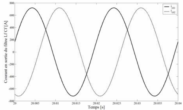
Fig. 6.44. Courants i_{ch1} , i_{ch2} .
